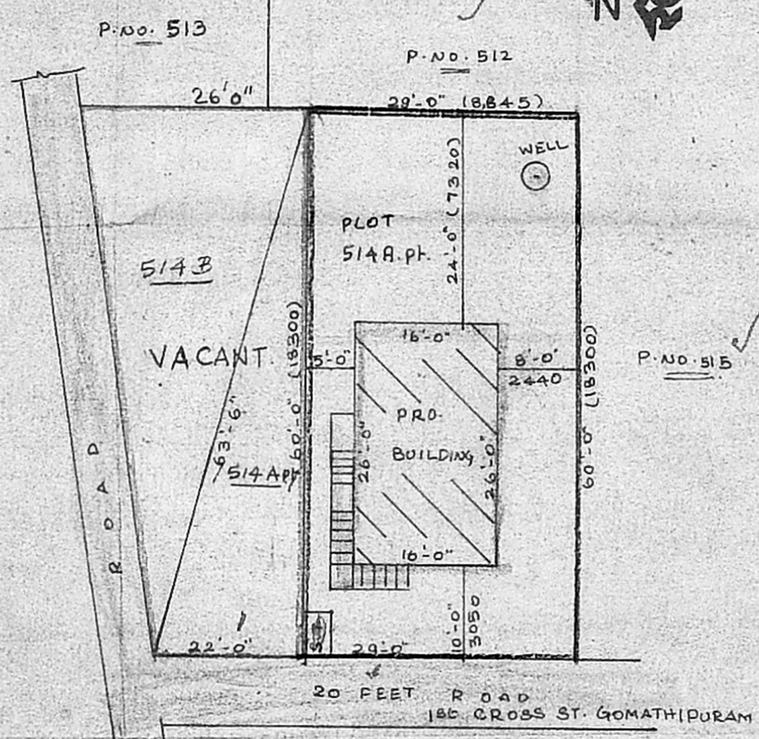
SITE PLAN SCALE 1:16
